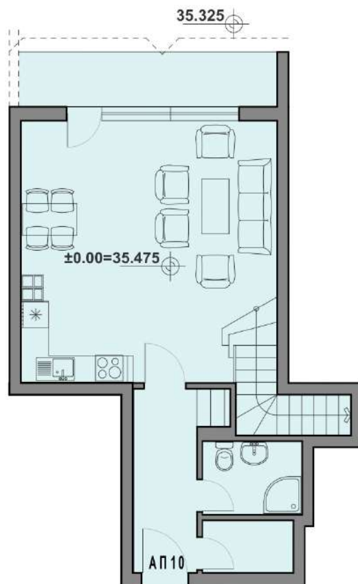
ЕТАЖ 1
