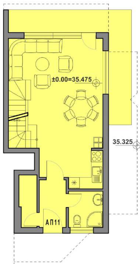
ЕТАЖ 1
