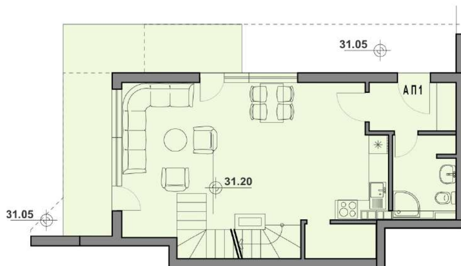
ЕТАЖ 1
